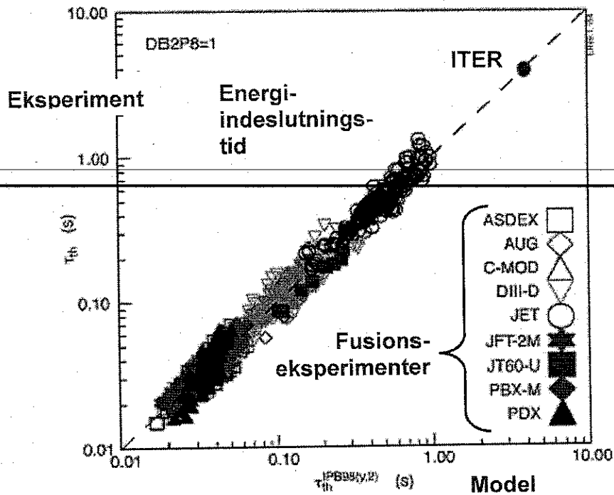
Figur 3 For alle typer plasmaer på en række fusionseksperimenter, store som små, er målte værdier af energi-indeslutningstiden plottet imod værdier beregnet ved hjælp af en og samme matematiske model. Det ses at model-beregningerne er i fin overensstemmelse med målte værdier. Model-beregningen bruges til forudsigelse af energi-indeslutningstiden i ITER.
